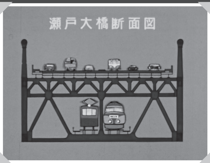
鉄道・道路併用橋の瀬戸大橋断面図
